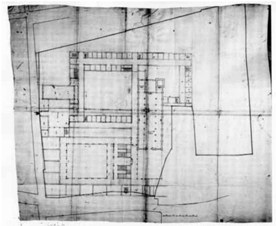
157. Mailand, Collegio di Brera, Plan Nr. 10.
