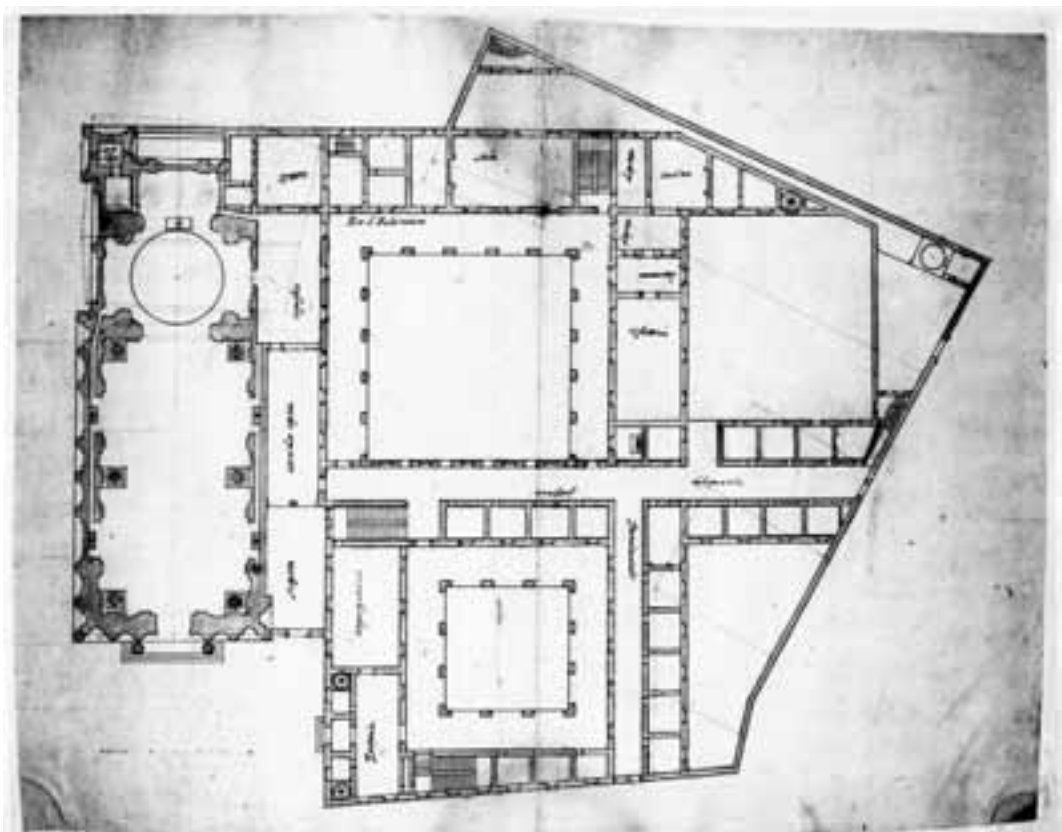
149. Mailand, Professhaus, Plan Nr. 19.
