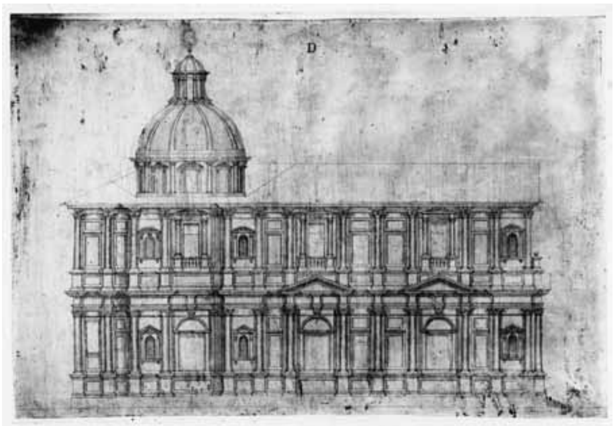
146. Mailand, S. Fedele, Plan Nr. 14 (Seitenprospekt).
