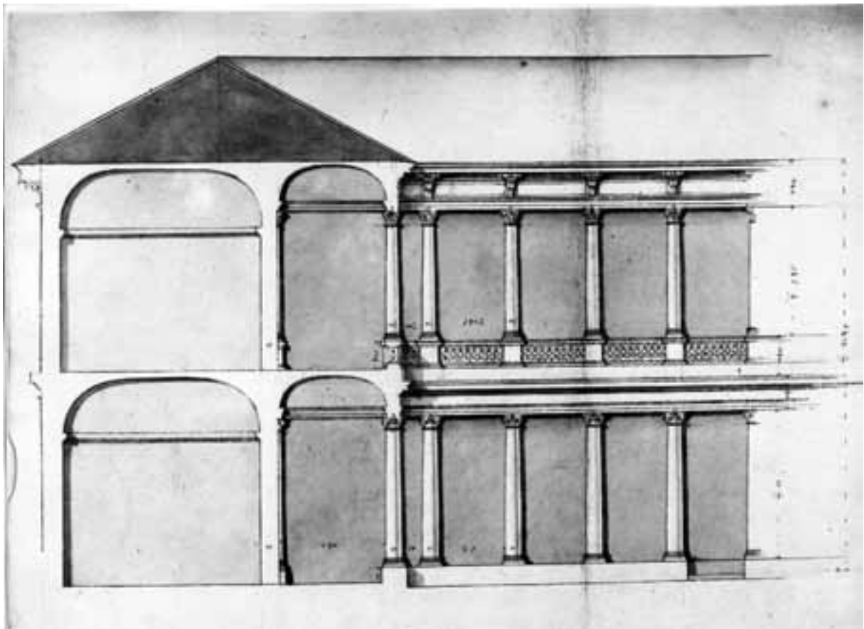
161. Mailand, Collegio di Brera, Plan Nr. 17.
