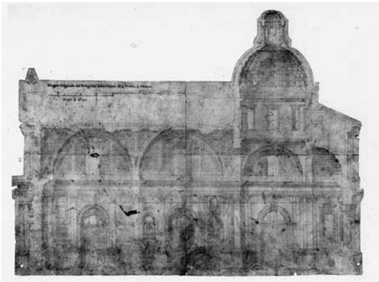
142. Mailand, S. Fedele, Plan Nr. 2 (Längsschnitt eines Vorentwurfs mit kassettierten Kreuzgewölben).
