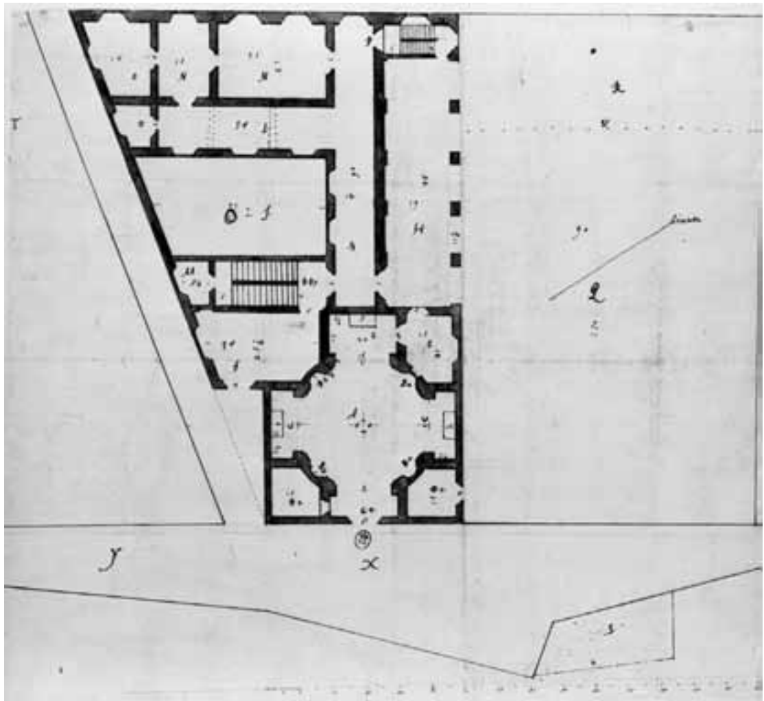
135. Genua, Albaro Residenz, Plan Nr. 2.
