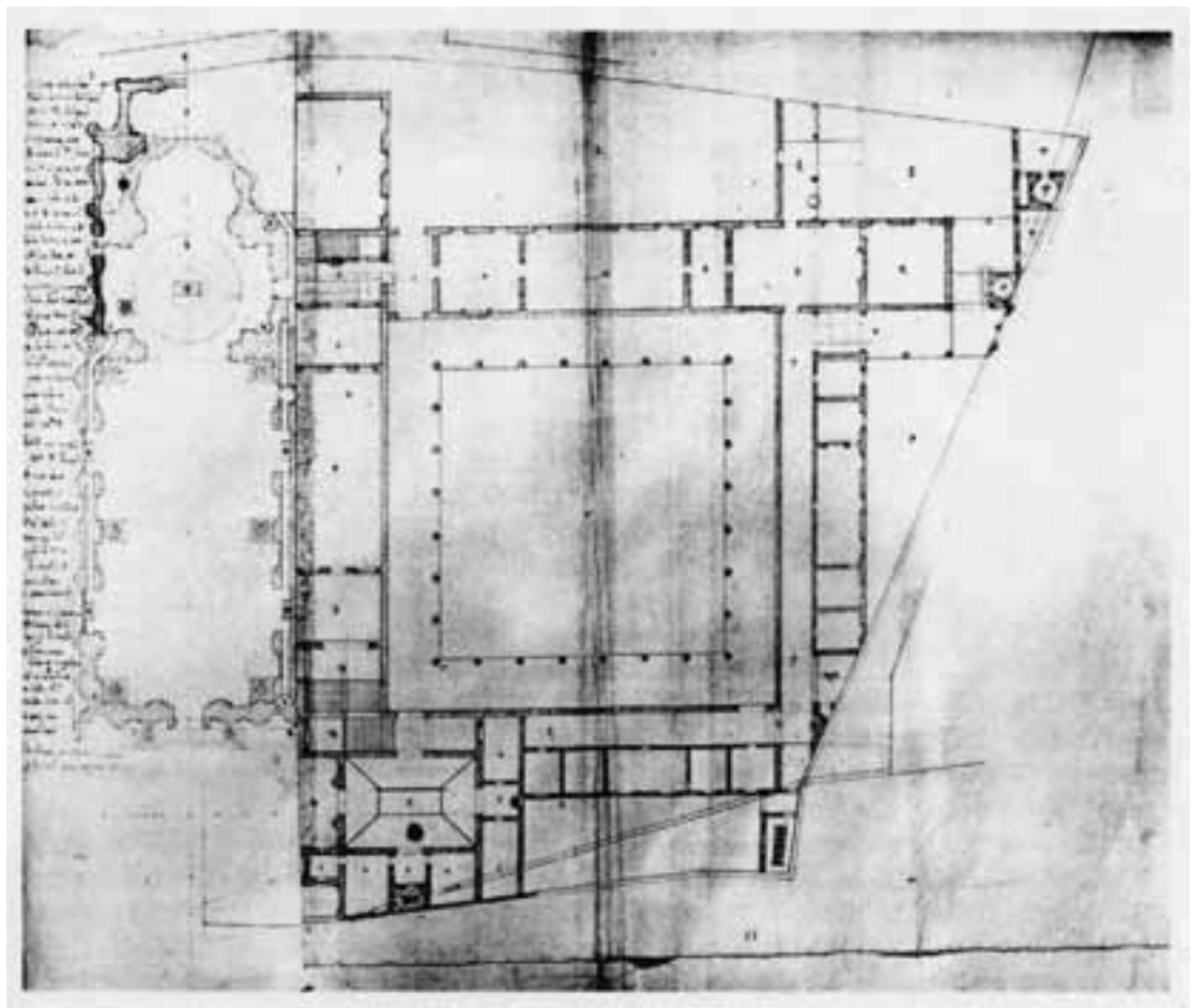
147. Mailand, Professhaus, Plan Nr. 17.
