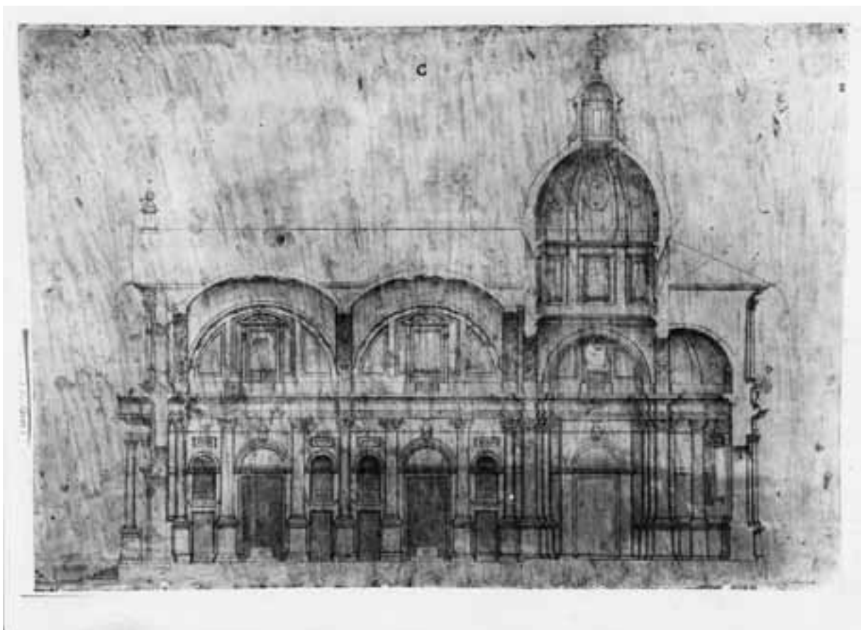
143. Mailand, S. Fedele, Plan Nr. 15 (Längsschnitt mit Stutzkuppelgewölben).
